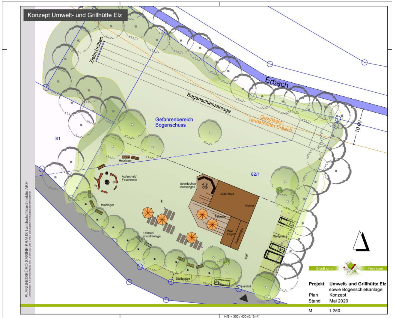
Abbildung 7: Planungskonzept, Kraus 05/2020
